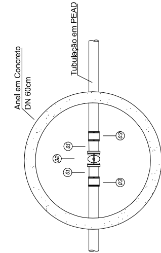
PLANTA BAIXA
