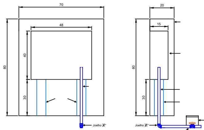
DETALHAMENTO MURETA COM UMA LIGAÇÃO DE ÁGUA
