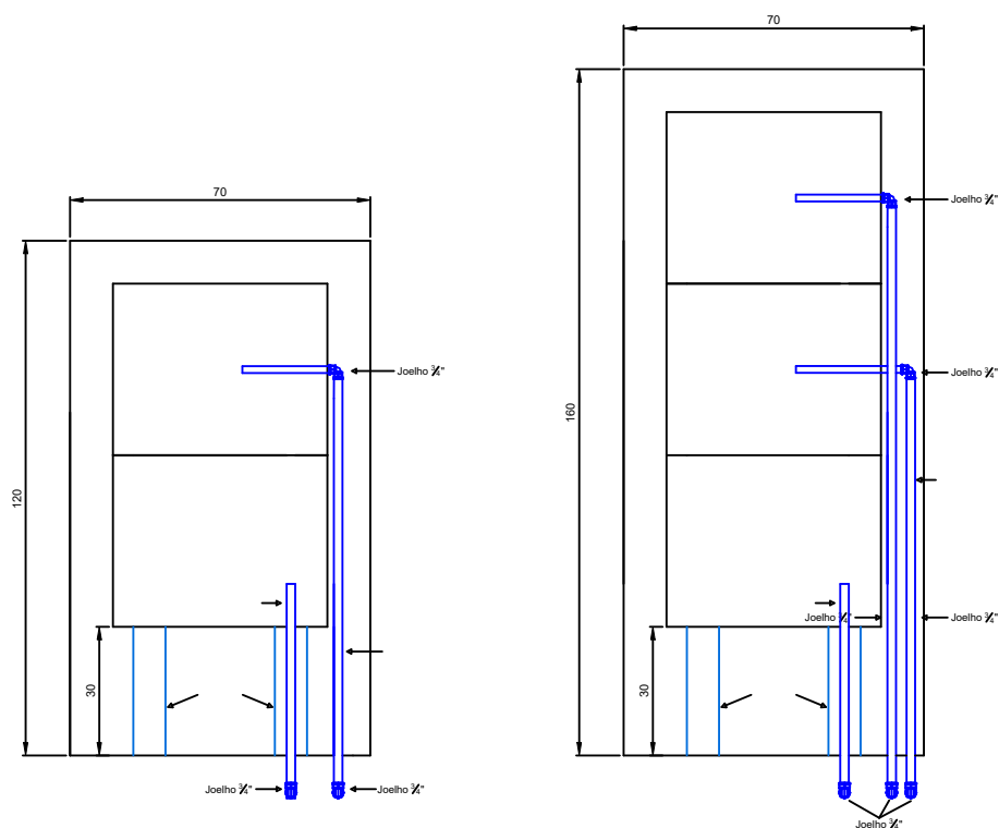
DETALHAMENTO MURETA COM DUAS E TRÊS LIGAÇÕES DE ÁGUA
